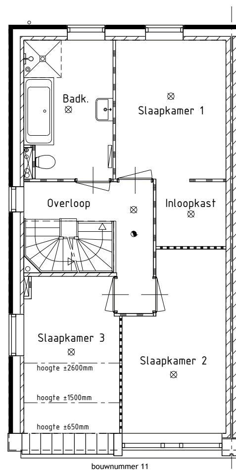
1ste Verdieping
